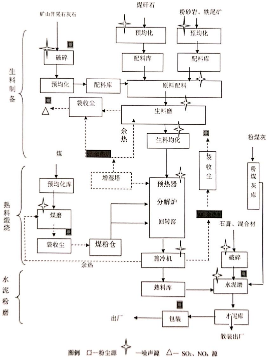
附件 2 水泥生产工艺流程图、污染源分布图
